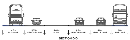
SECTION D-D
